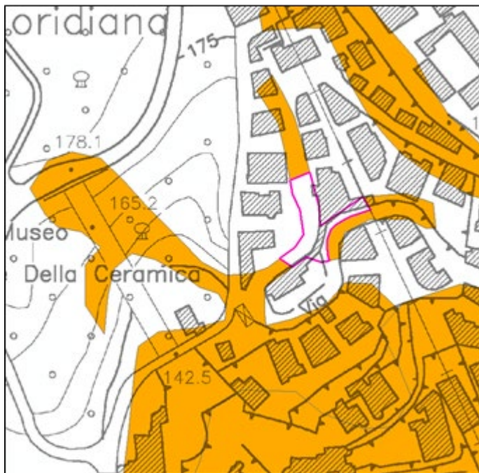
STRALCIO DEL PSAI – CARTA DEL RISCHIO DA FRANA CON MODIFICA
